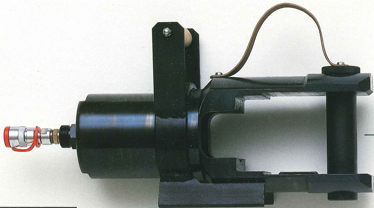
Presshuvud V 1470 Vikt: 21,5 kg. Inkl låda 28,5 kg.
